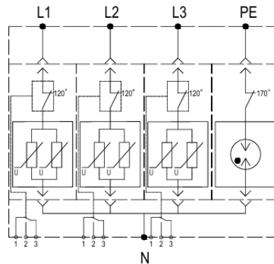
Принципиальная схема
